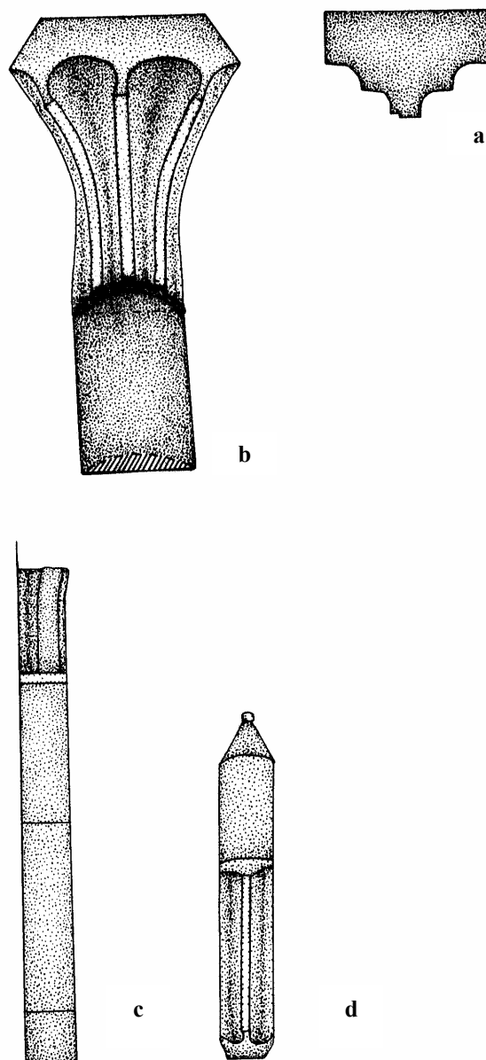
Fig. 4 – Benic. Biserica reformată. Detalii: a. ancadrament de fereastră – latura de sud-vest a corului; b. mănunchi de trei nervuri la semicolonetele ce delimitează cele două travee ale corului ; c. semicolonetă angajată, latura de nord-est a corului; d. consolă – colțul de nord-vest al corului
